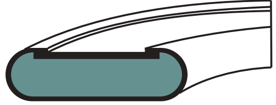
Çift Ceketli Conta Kesiti
